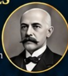
H. BECQUEREL (1896)
