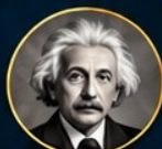
ALBERT EINSTEIN (1905)
